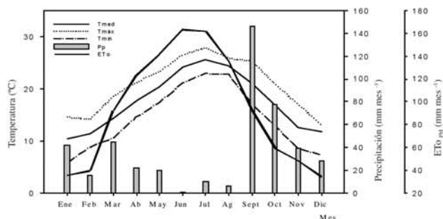
Figura 9. Evolución media mensual de la temperatura máxima (Tmáx °C), mínima (Tmin °C), media (Tmed °C), evapotranspiración de referencia (ETo mm mes -1 ) y precipitación (Pp, mm mes -1 ) durante el periodo 2006-2009 en Cartagena (cultivo de almendro).
