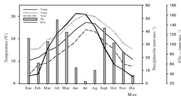
Figura 8. Evolución media mensual de la temperatura máxima (Tmáx °C), mínima (Tmin °C), media (Tmed °C), evapotranspiración de referencia (ETo mm mes⁻¹) y precipitación (Pp, mm mes⁻¹) durante el periodo 2006-2009 en Molina de Segura (cultivo de nectarino).
