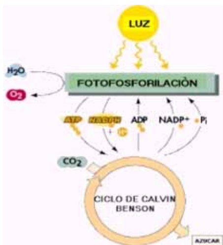
Figura 2. Esquema de la fotosíntesis.
